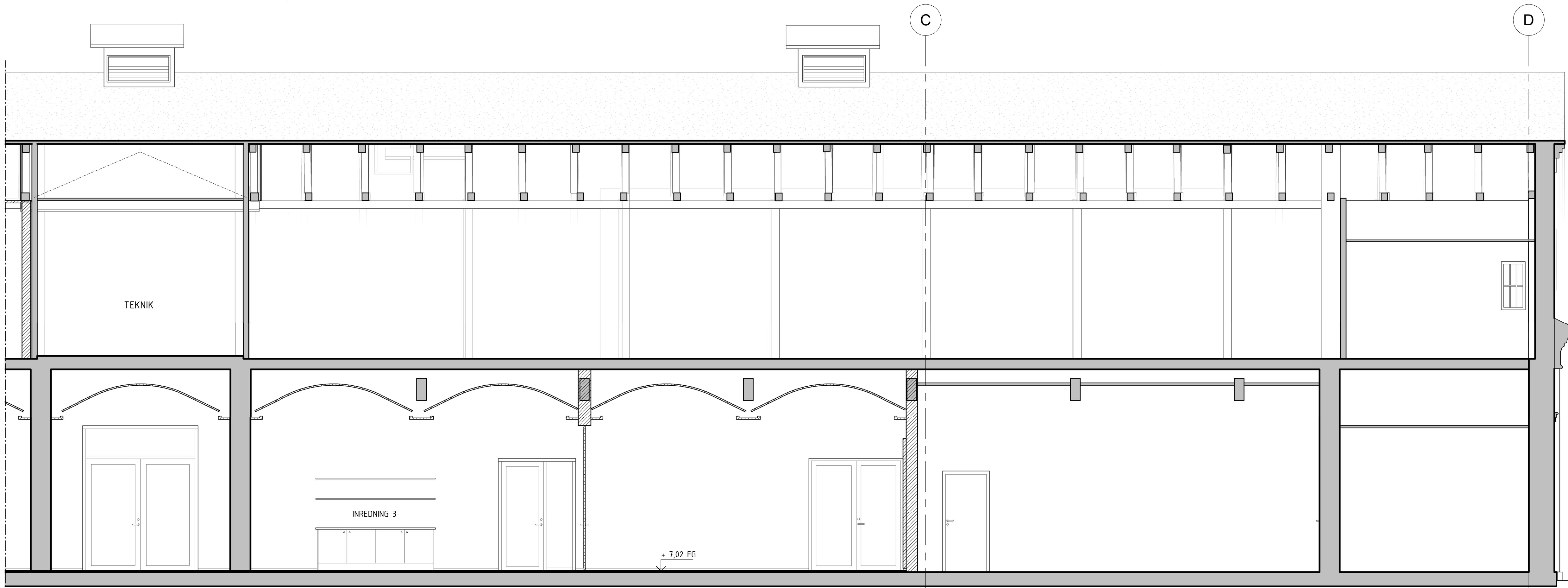
SEKTION D-D (DEL 1)
