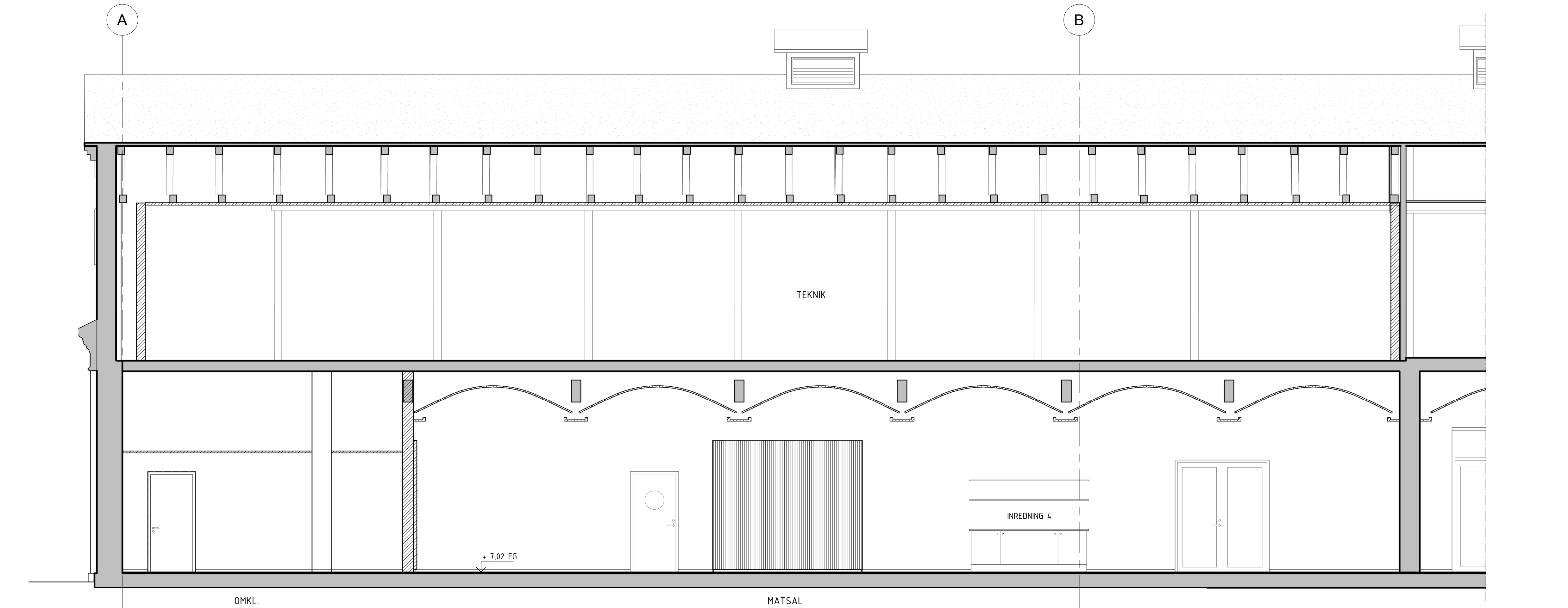
SEKTION D-D (DEL 1)
